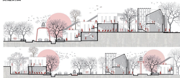
街道剖面
